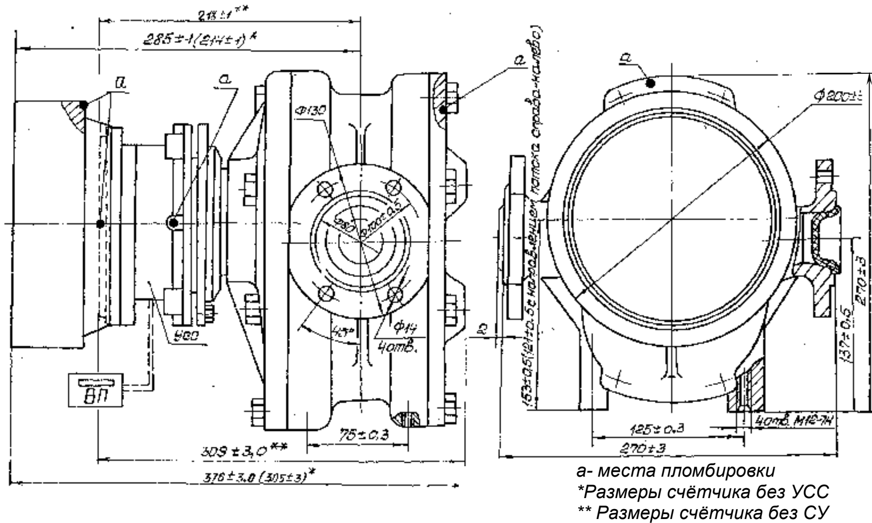
Рисунок В1. Счётчик жидкости с овальными шестернями унифицированный; ППО-40-0,6 СУ; ППО-40-0,6 СУ-01 Габаритные и присоединительные размеры
